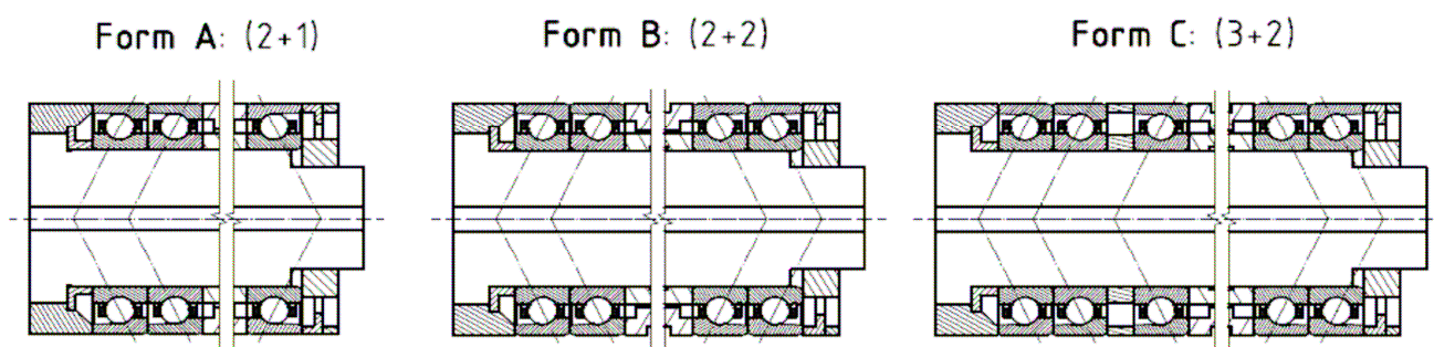
Bauformen von Kurzspindeln
